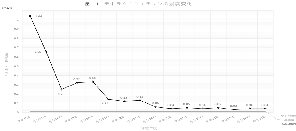
▲ 図-1 汚染除去経過グラフ
