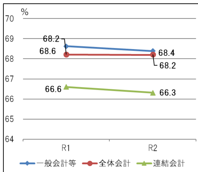
老朽化比率
