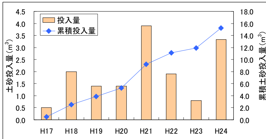
一宮海岸の養浜実績
